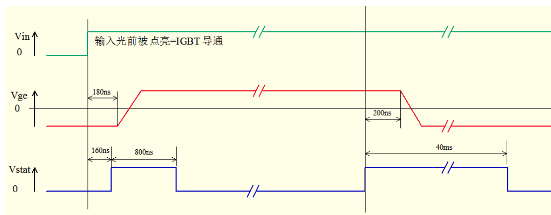
TPH836-65S 高压驱动板故障时序
