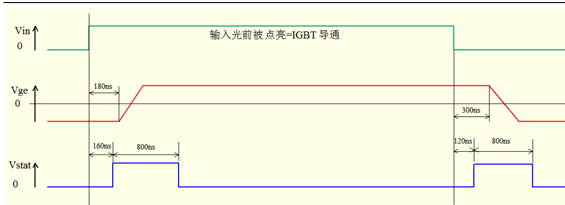
TPH836-65S 高压驱动板工作时序
