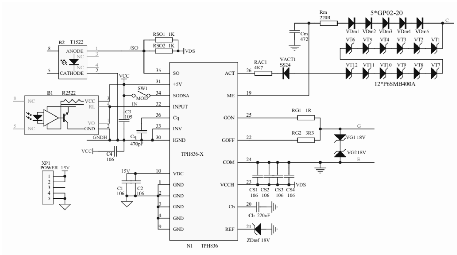
TPH836-65S 电路原理图
