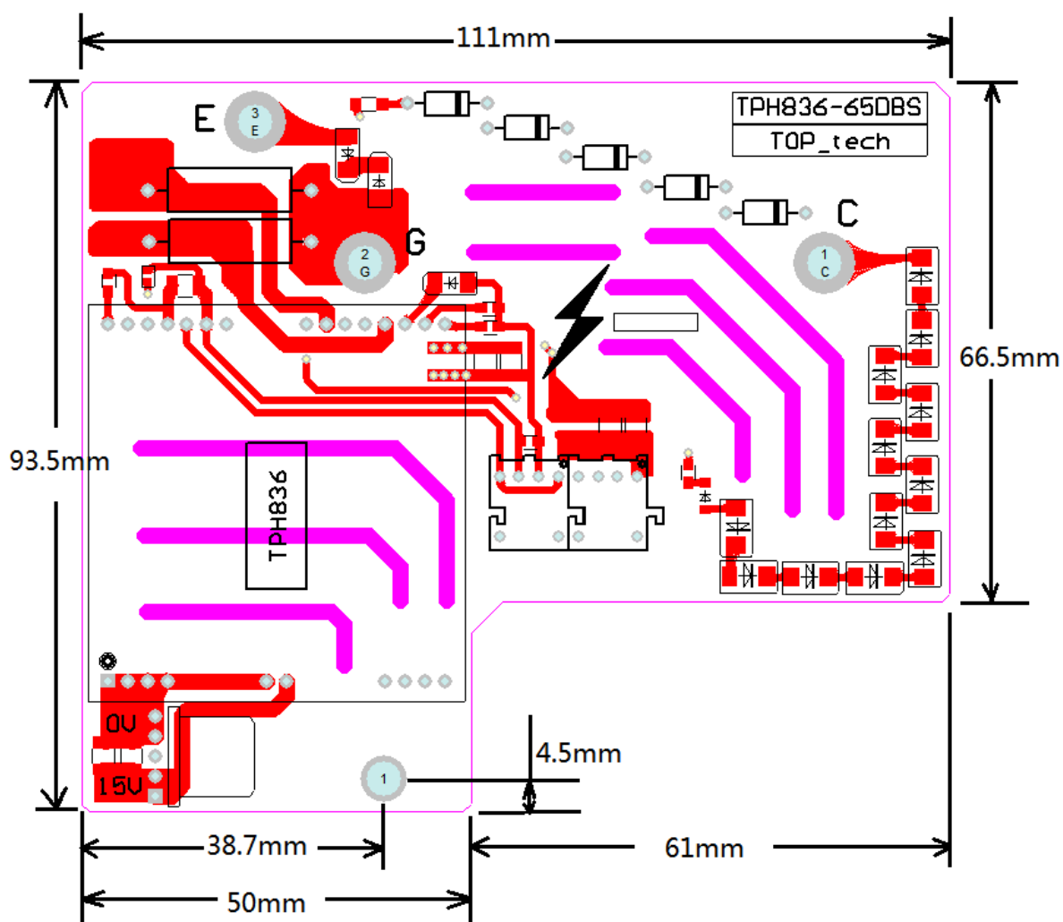
TPH836-65S 机械尺寸图
