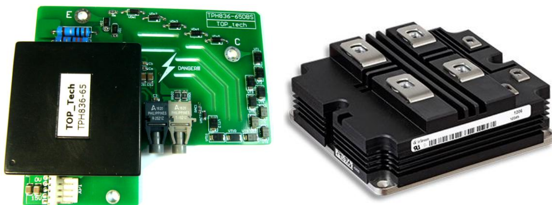
TPH836-65S 驱动板和所对应的 IGBT 模块外形图
